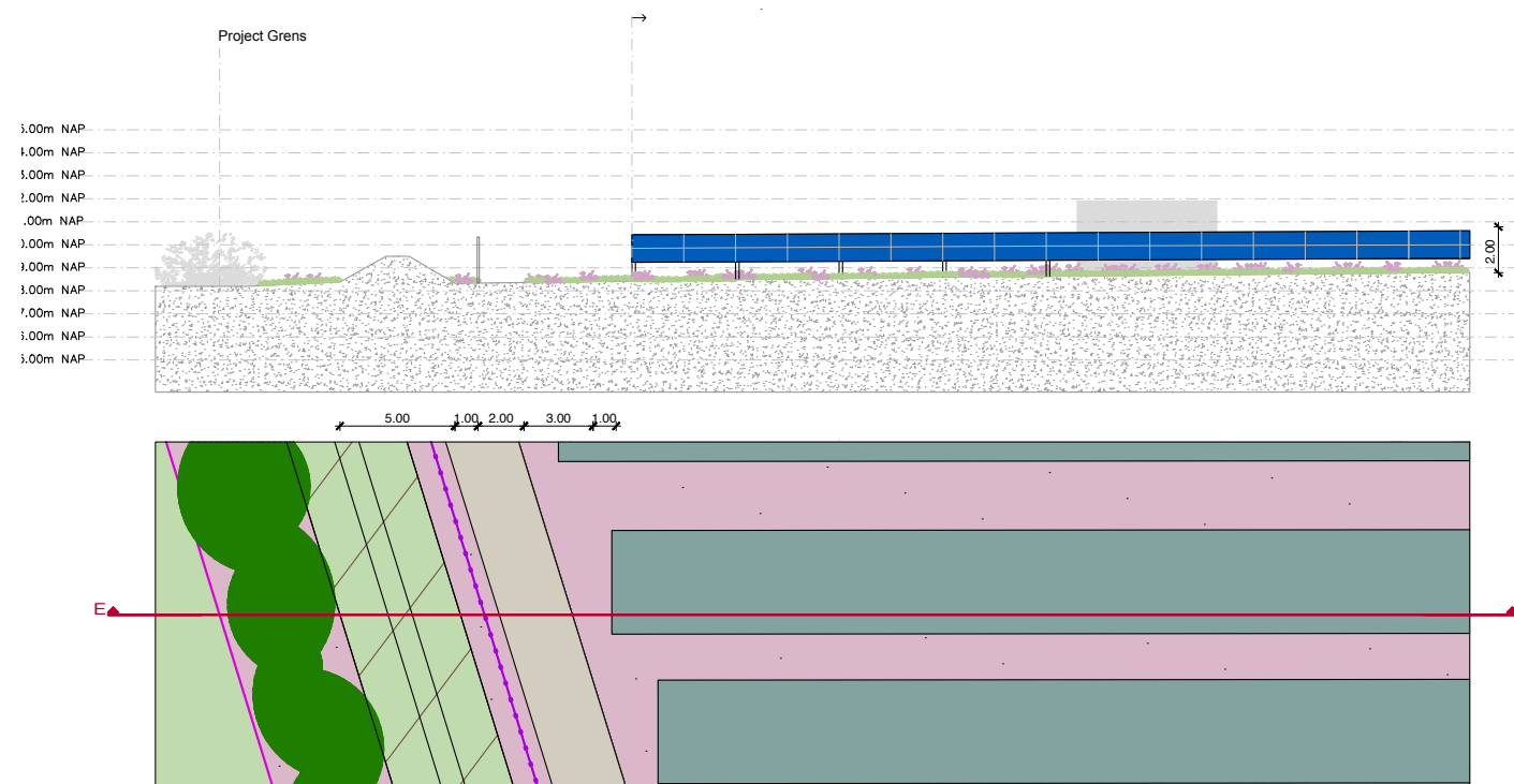
Doorsnede EE
